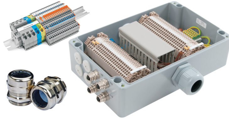
Kundenspezifische Bestückung, Klemmleisten und Verteilergehäuse
