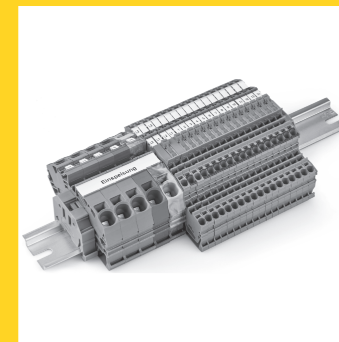
Klemmenleisten nach Wunsch
