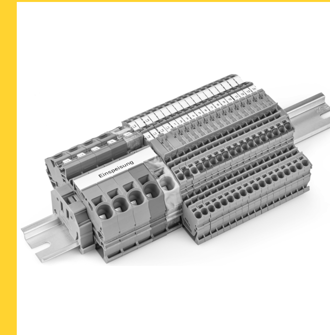
Klemmenleisten nach Wunsch
