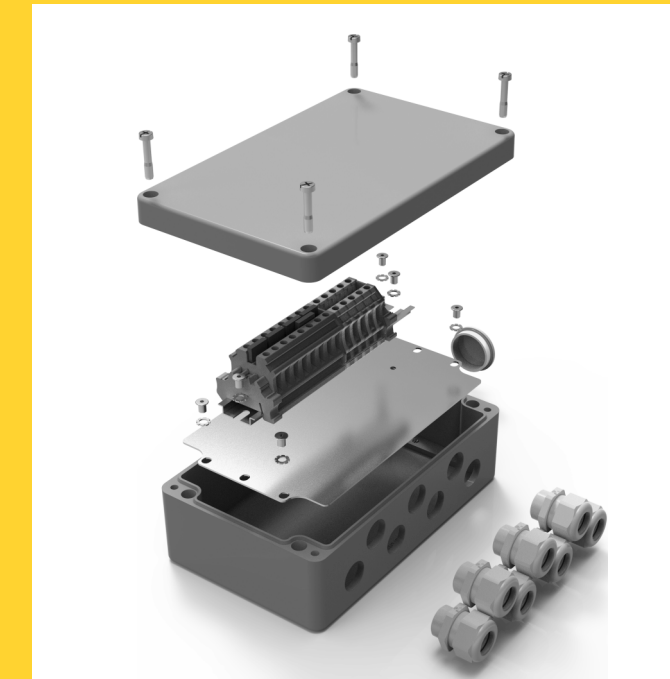
Komplett vormontiertes Gehäuse
