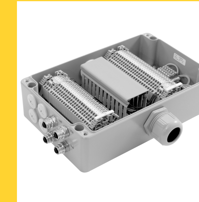
Kundenlösung Verteilergehäuse
